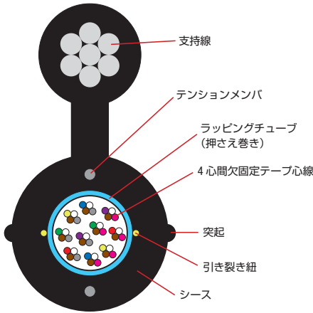
<40心構造>
